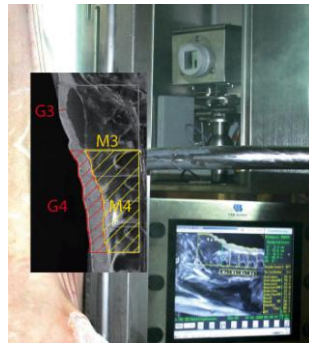
Figure 2 : un scanner RX permet de différencier dans le volume trois tissus des carcasses et pièces de porc : le muscle, le tissu gras et l'os
